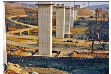
Bauarbeiten an der Großbrücke über die Flöha im Jahr 1990. Die Pfeiler sind fast fertiggestellt, der darauffolgende Vorschub Überbau begann im Januar 1991. Da war der Überbau an der Großbrücke über den Hetzbach bereits abgeschlossen. Im Vordergrund das Gleis der Bahnstrecke nach Olbernhau-Grünthal.
