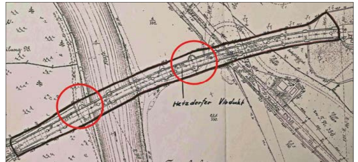
Lageskizze des Hetzdorfer Viadukts. Farbig hervorgehoben sind die beiden Hauptpfeiler.
